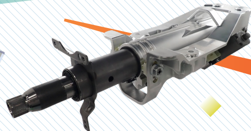
電動チルト&テレスコピック ステアリングコラム
